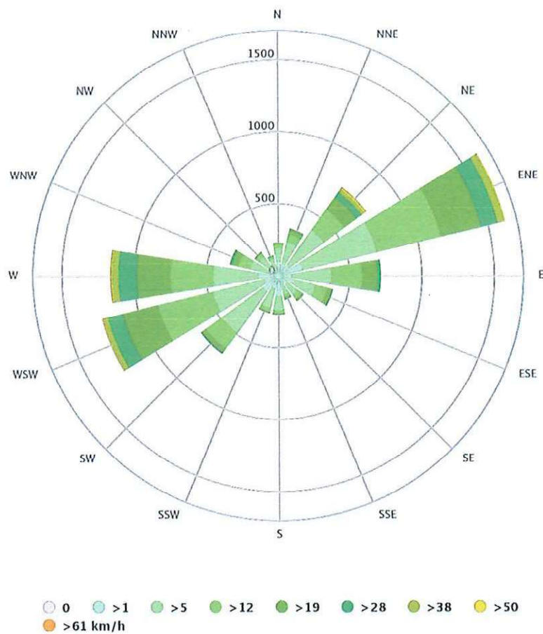
Direcția predominantă a vânturilor Alexandria
