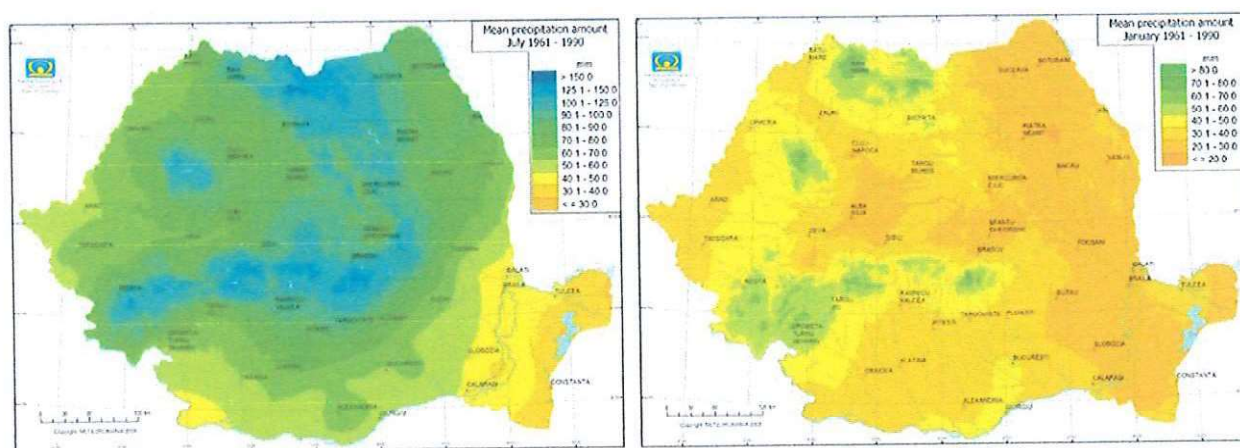
Precipitații medii lunare multianuale *sursa INMH
